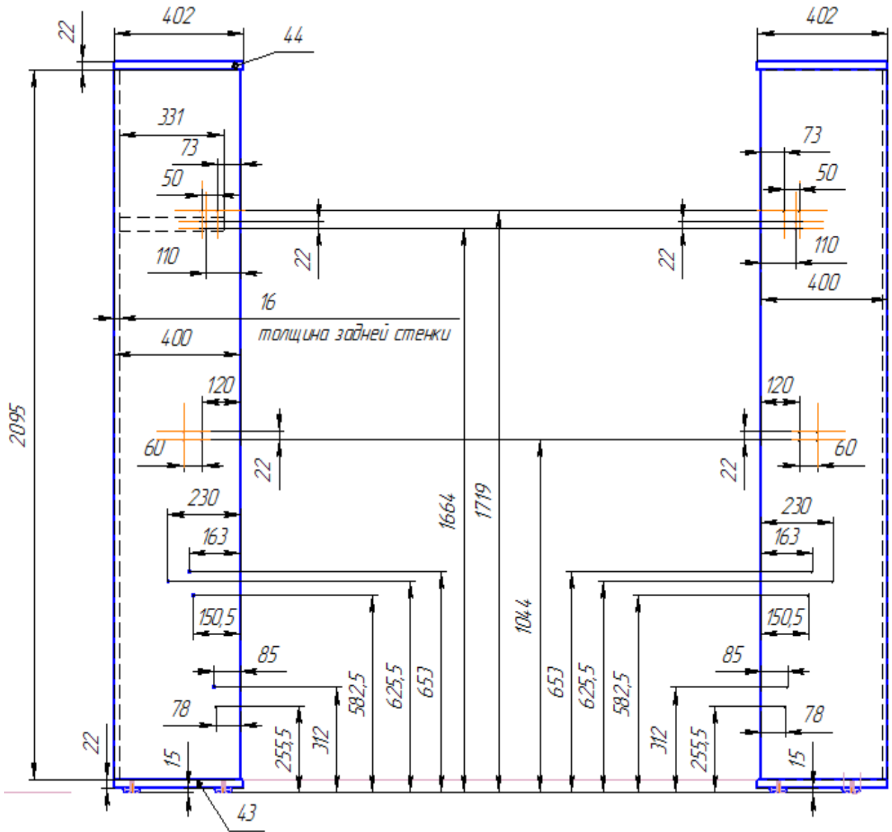
БОКОВИНА ЛЕВАЯ
